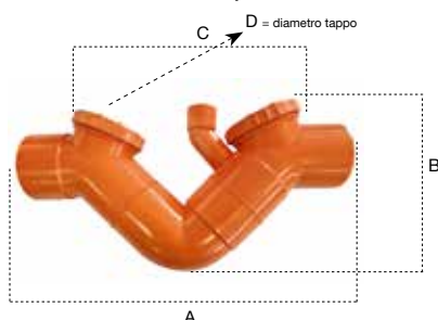
VENT SIPHON - 2 caps
